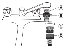
Filetages Internes
